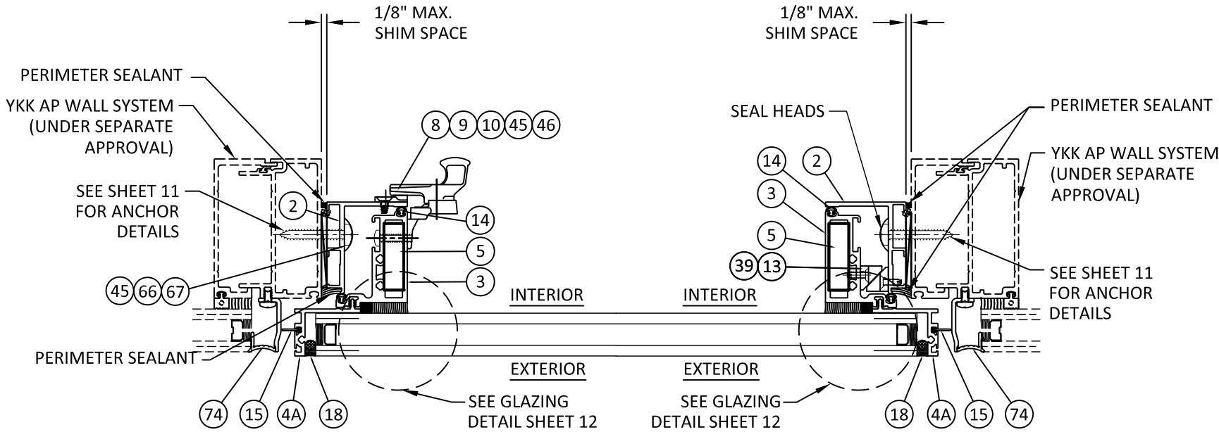
X-10 HORIZONTAL SECTION LOCK JAMB - HINGE JAMB YWW 50 / 60 TU - SSG
